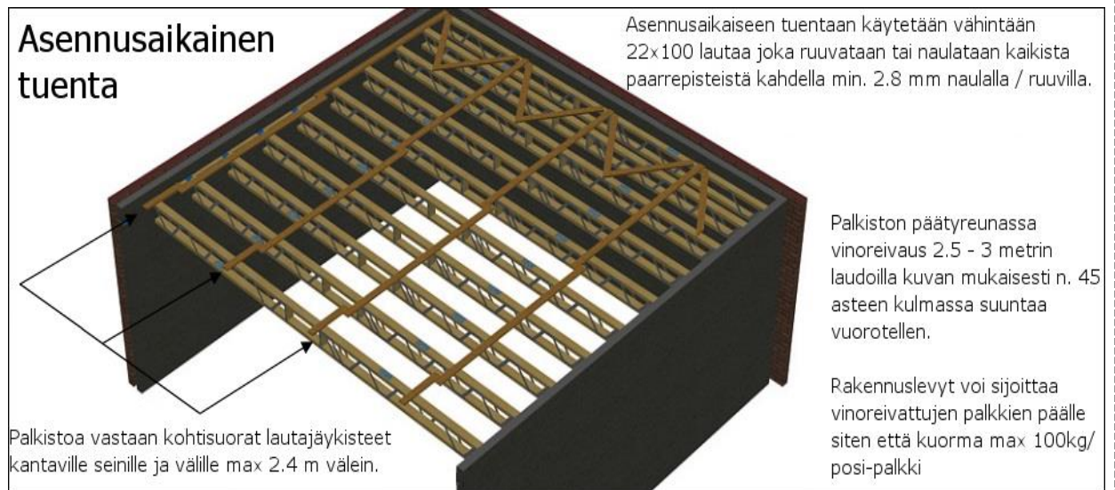
KUVA 4 AENNNUSAIKAINEN TUENTA
