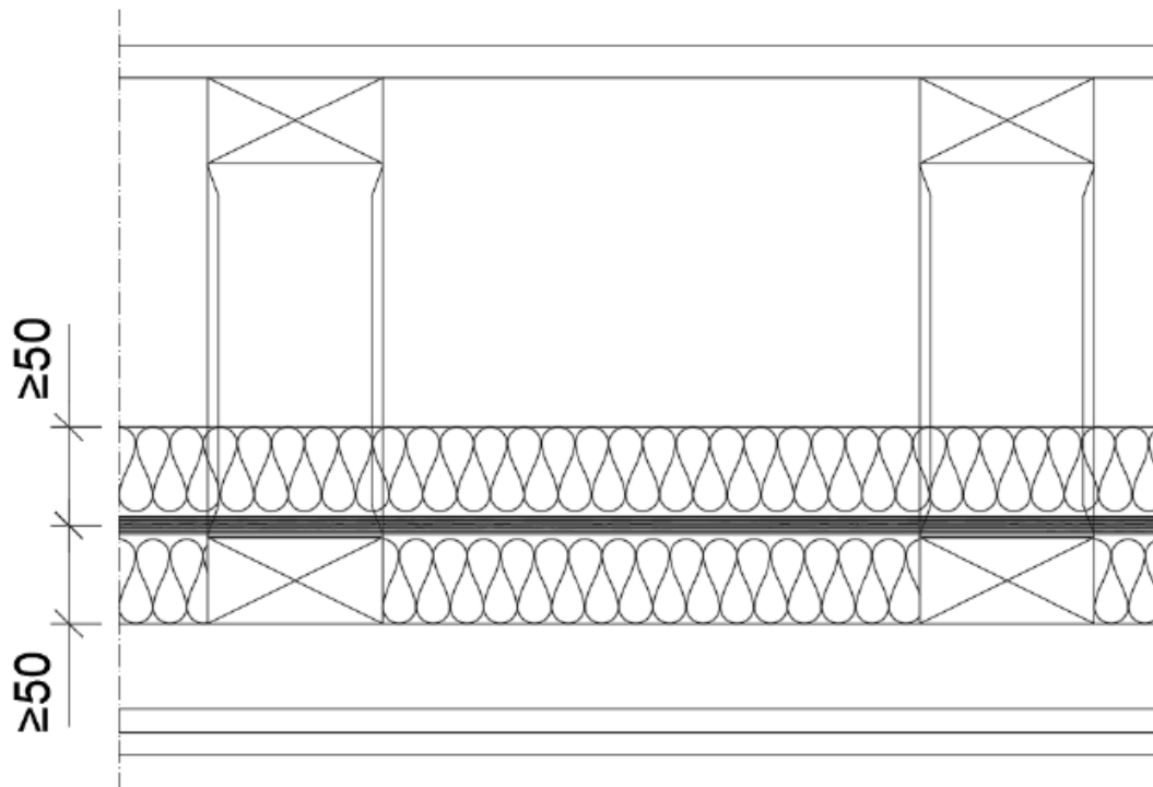
KUVA 12 SÄHKÖJOHTOJEN SUOJAUS ONTELOTILASSA
