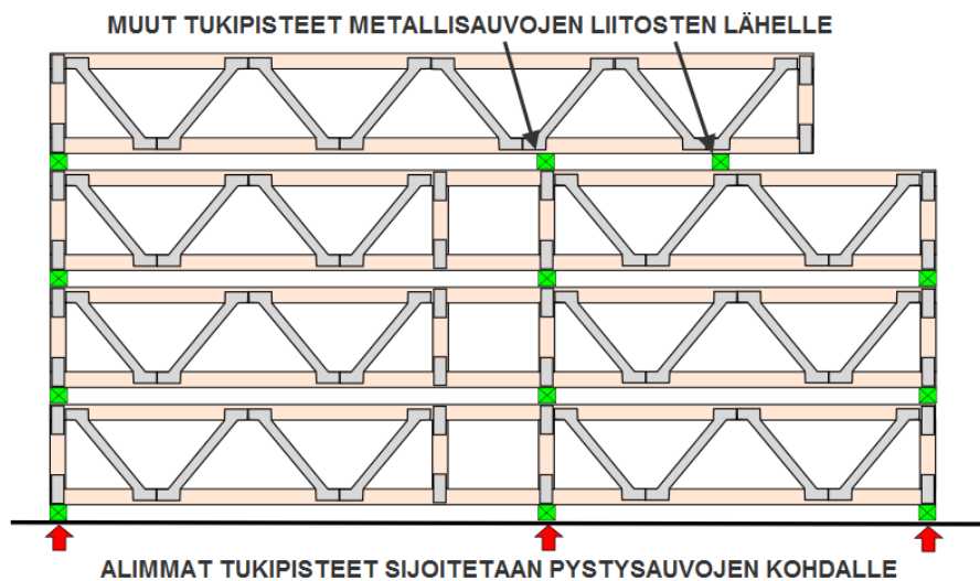
KUVA 1 PALKKIEN VARASTOINTI
